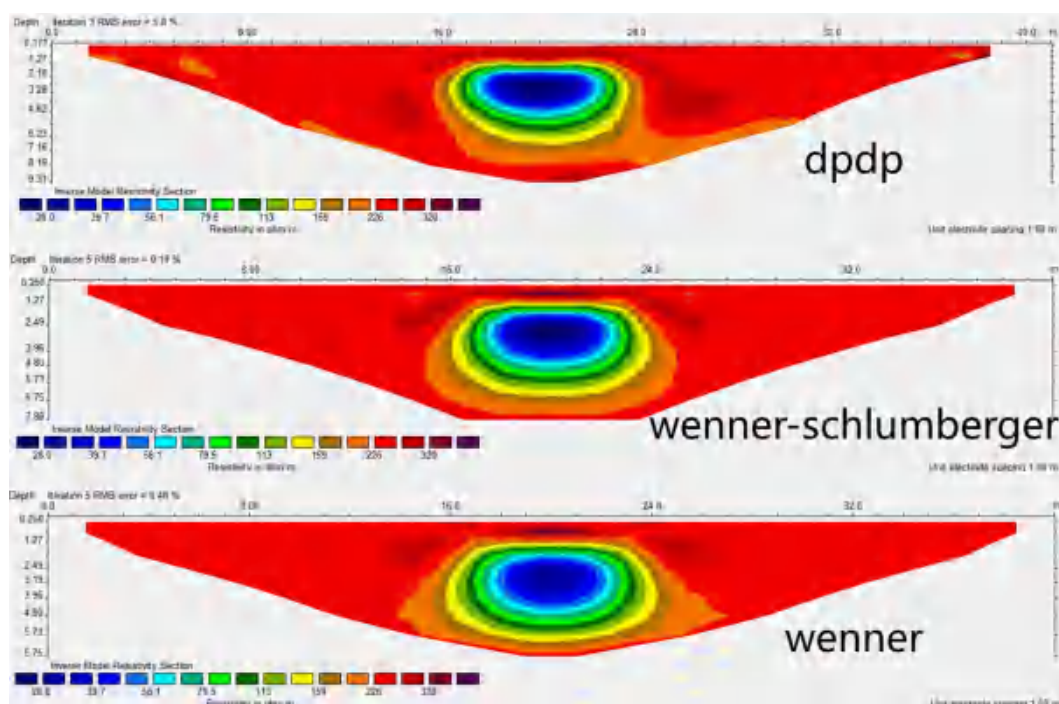
图 14 不同 ERT 装置对地下含水空洞低阻异常体的反演成像对比
