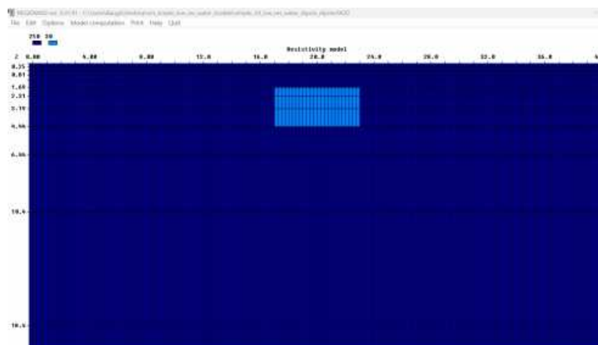
图 13 ERT 探测地下含水空洞的二维电阻率模型
